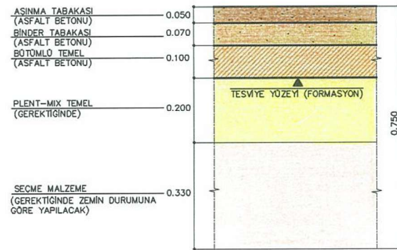
MEVCUT ASFALT KAPLAMALI YÜZEYLERDE UYGULANACAK ÜST YAPI TİP ENKESİTİ
