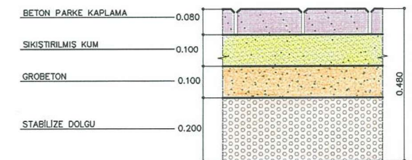
TRETUVAR ÜST YAPI KALINLIKLARI
