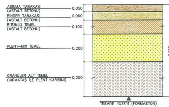
ALT GEÇİTTE UYGULANACAK ÜST YAPI TİP ENKESİTİ
